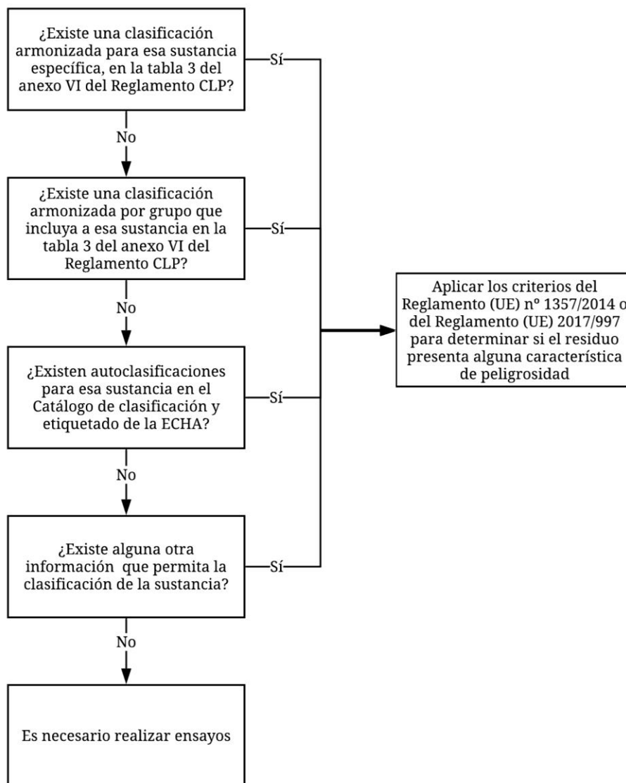
Figura 8. Diagrama de flujo del proceso de clasificación de un residuo a partir de la clasificación de las sustancias que contiene
