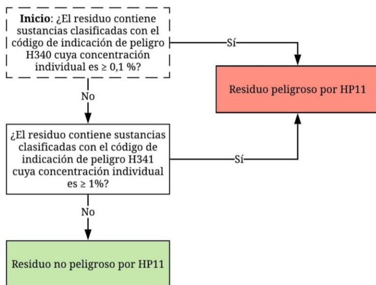
Figura 19. Diagrama de flujo para la evaluación de la característica de peligrosidad HP 11
